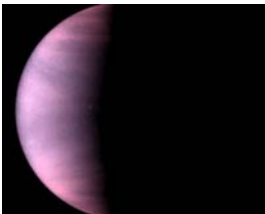
Venus Hubblesite 1995
